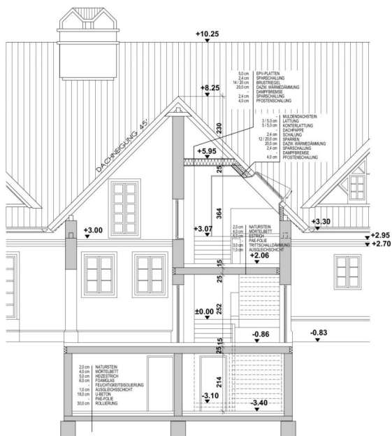
WH / SCHNITT G - G
