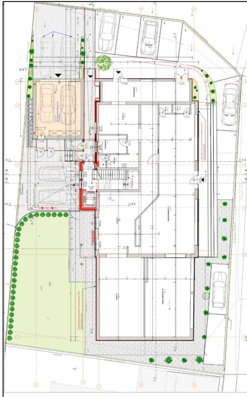
Top 1 Erdgeschoß und Aussenbereich
