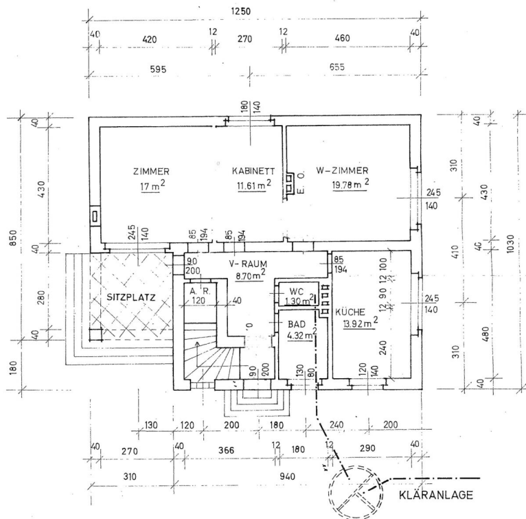
ERDGESCHOSS M 1:100
