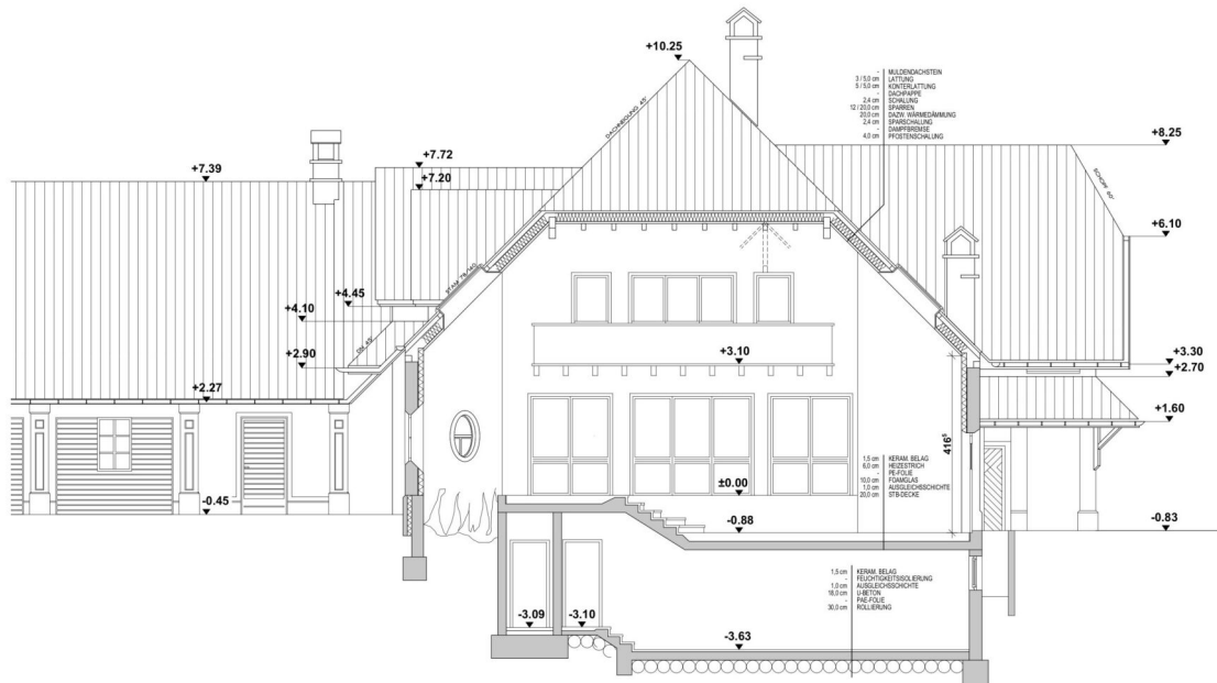
WH / SCHNITT F - F
