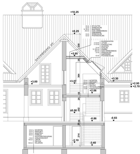
WH / SCHNITT G - G
