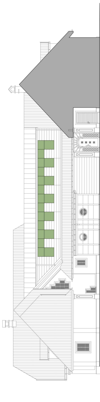
BÜRO ANSICHT v. OSTEN - HOF
