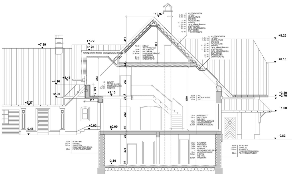
WH / SCHNITT E - E
