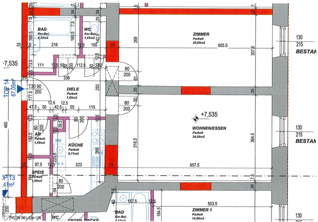
TOP 14 2.OG BESTANDSOBJEKT ca.67,05m 2 / ca. 15,1m 2 Terrasse
