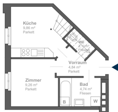
OG 3_M 1:100
