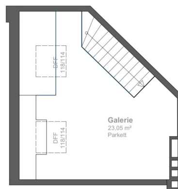
Galerie_M 1:100
