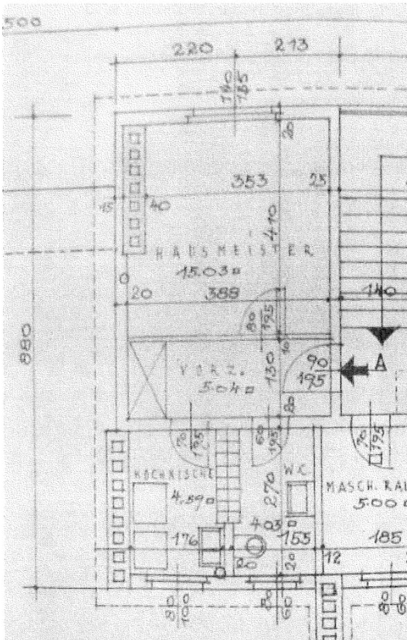
W19 Grundriss
