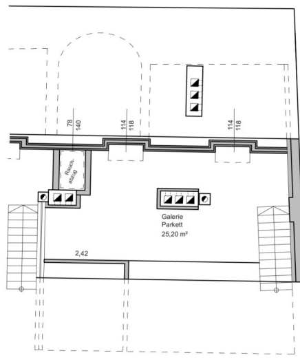
oberes Geschoss
