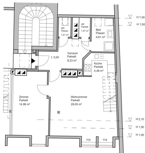
unteres Geschoss
