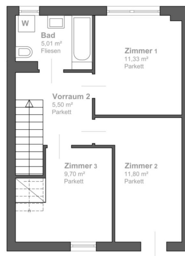
OG 1_M 1:100
