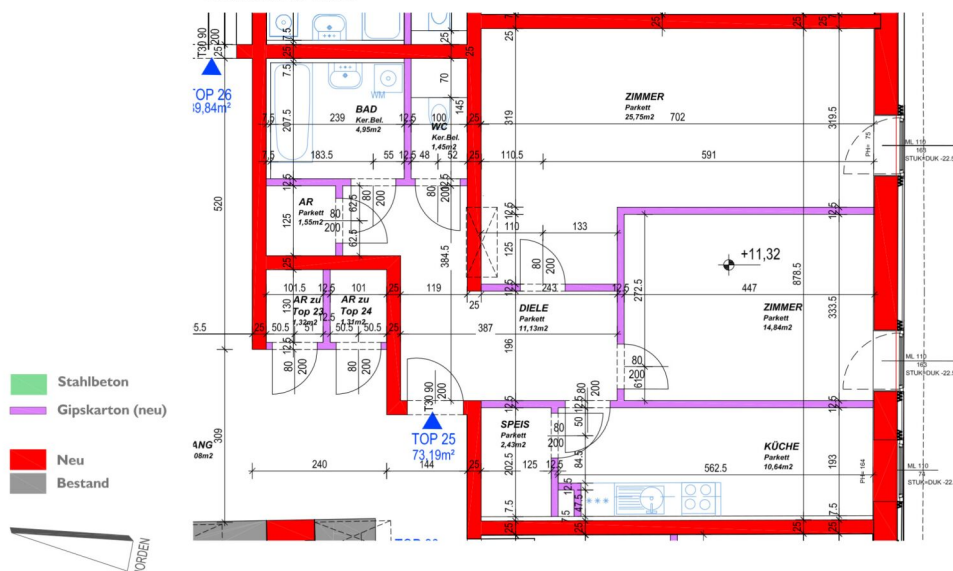
Grundriss M 1:100
