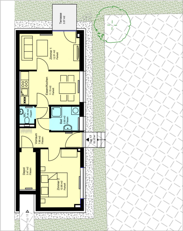
Top 17 - 1:100
