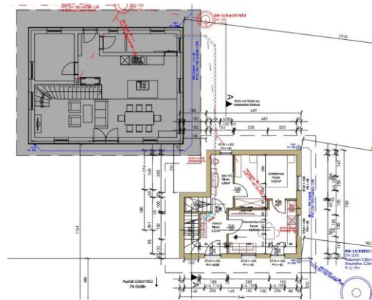
Plan Zubau Erdgeschoß
