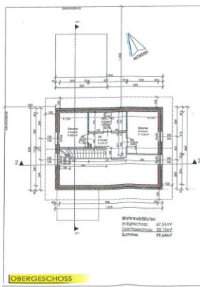
Plan Haupthaus Obergeschoß
