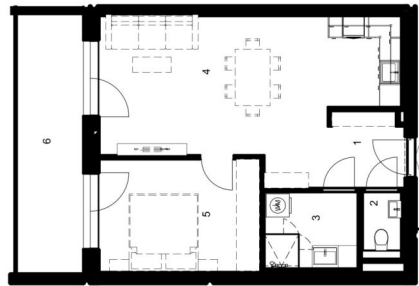
GRUNDRISS 2.OBERGESCHOSS
