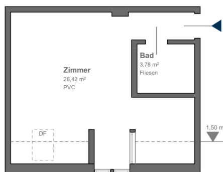
DG_M 1:100
