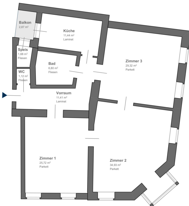
1.OG_M 1:100
