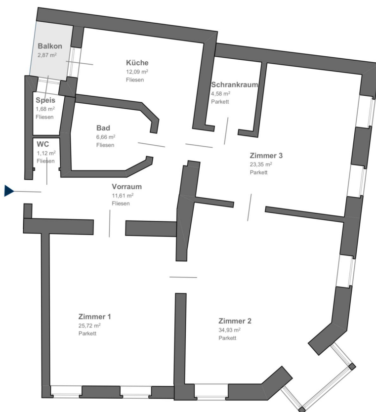
2.OG_M 1:100
