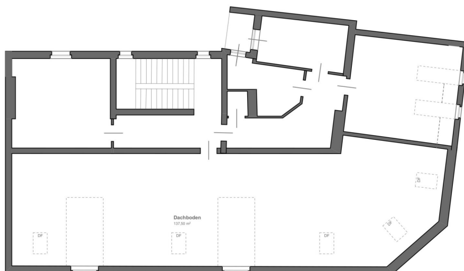
Keller_M 1:150
