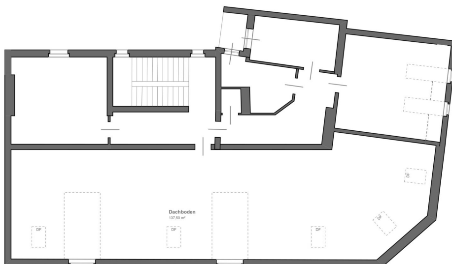
Keller_ M 1:150
