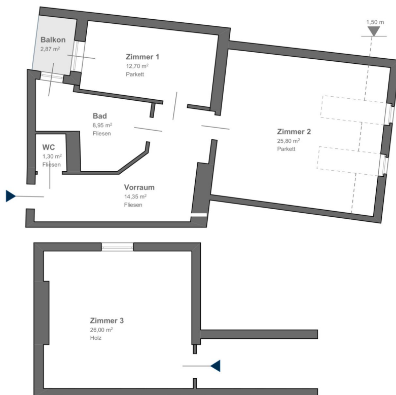
DG_M 1:100
